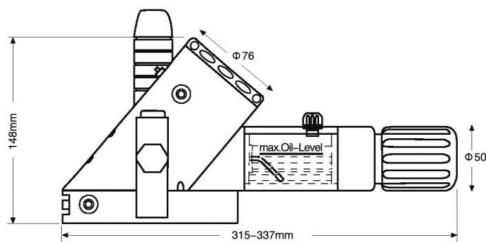
高压校验仪外形图纸
